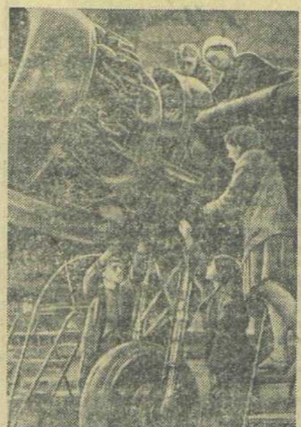
Молодая женщина-бригадир комсомолец Марины Богачевой на сборе бомбардировщиков. Она выполняет нормы на 300 прои. Это — передовая бригада девушек на 11-ом заводе. На снимке бригада за монтажом приборной группы самолёта.
